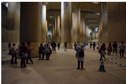
首都圏外郭放水路「調圧水槽」 （提供：江戸川河川事務所）
